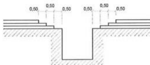
Átlapolásos technika
