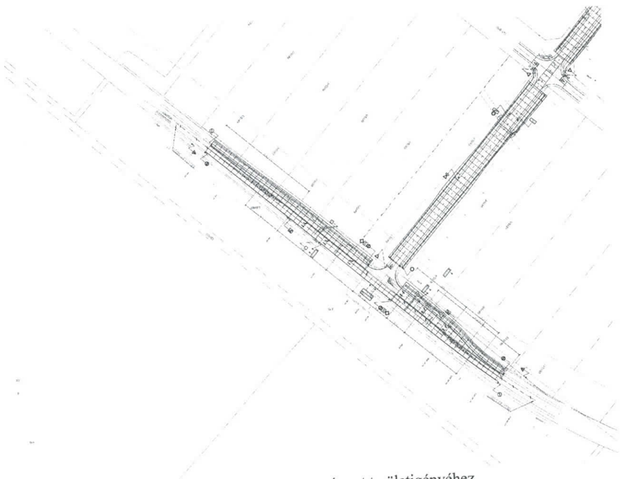
közlekedési vázlat a csomópont területigényéhez
